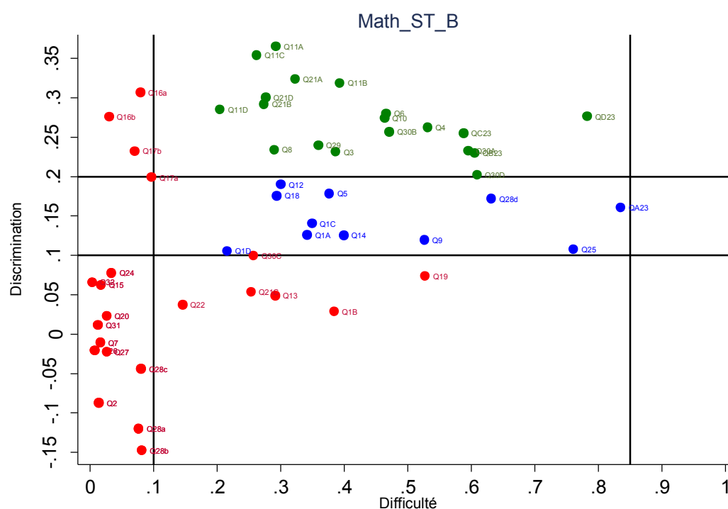
Graphique 1. Analyse des items du test B des mathématiques (troncs communs Sciences et Technique)
