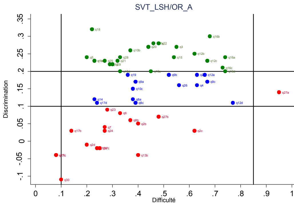
Graphique 4. Analyse des items du test A des Sciences de la Vie et la Terre (Lettres/Original)
