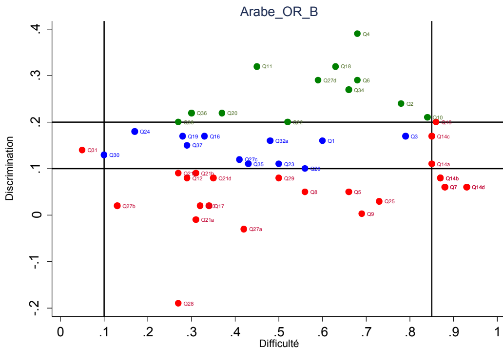
Graphique 7. Analyse des items du test A de la langue Arabe (Originel)
