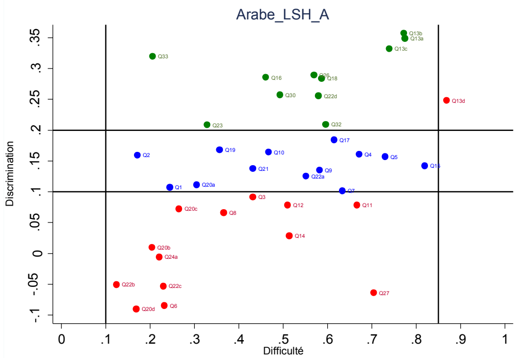
Graphique 6. Analyse des items du test A de la langue Arabe (Lettres et Sciences Humaines)
